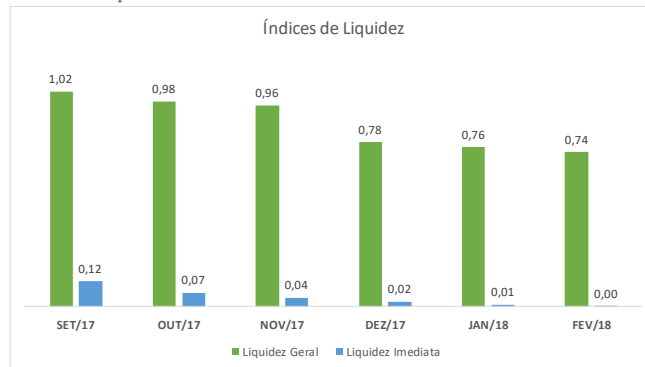
Gráfico 4 - Liquidez Corrente.
